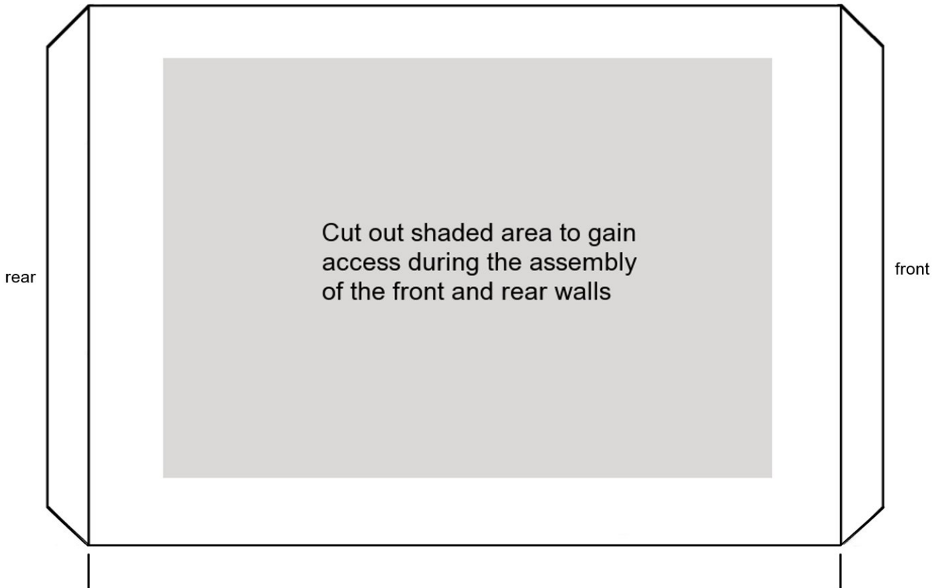
Baseplate
